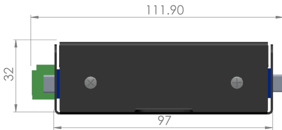
YAN GÖRÜNÜŞ
