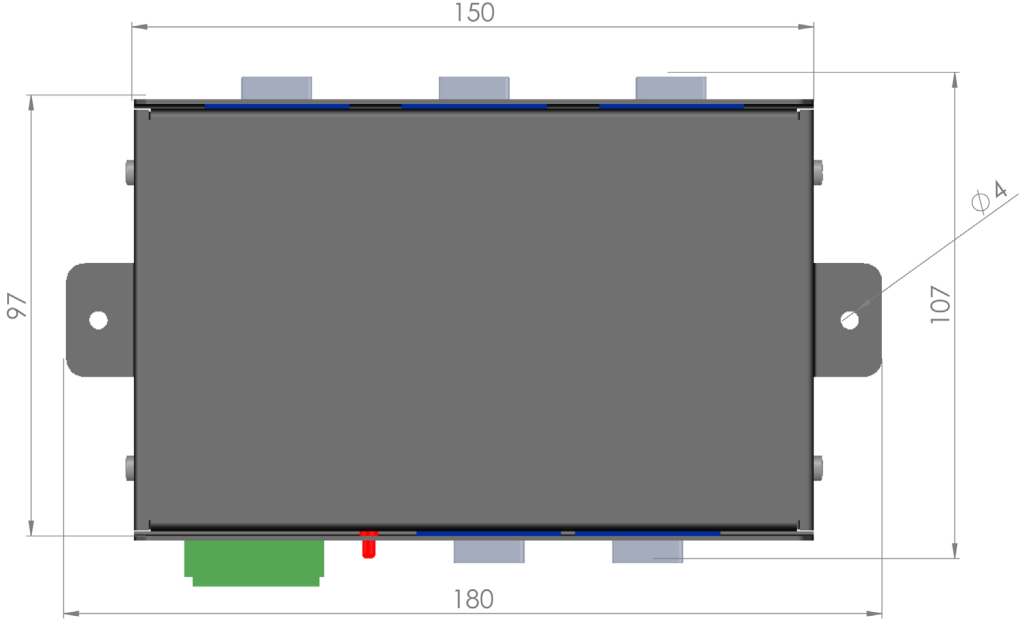
ÜST GÖRÜNÜŞ
